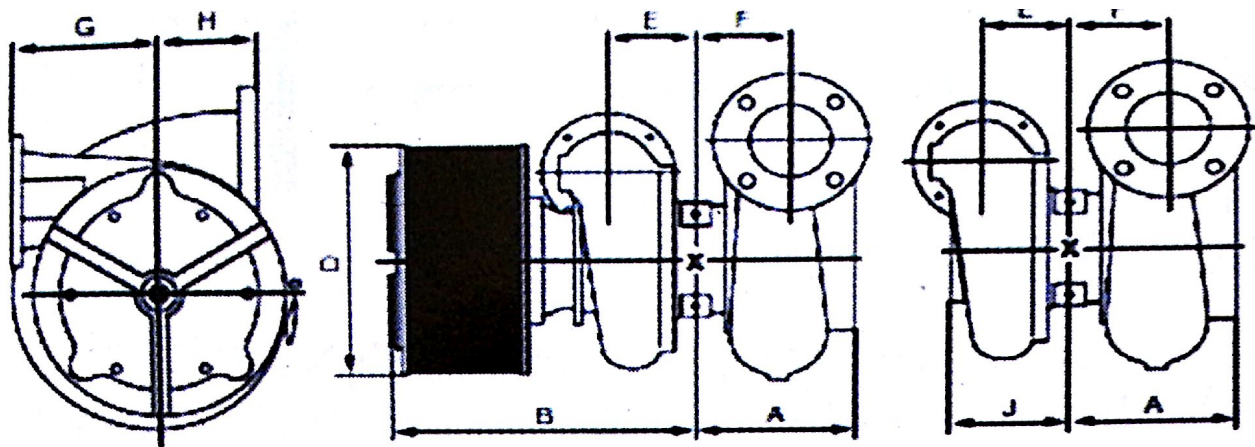
BF-J系列增压器 BF-J Series Supercharger
