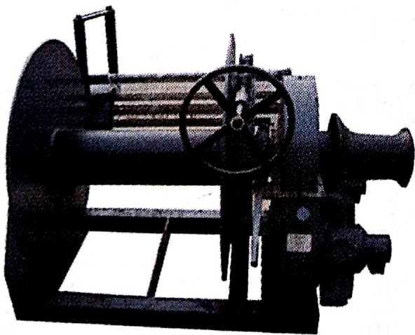
RQG6 液压卷纲机 Rope Reel
